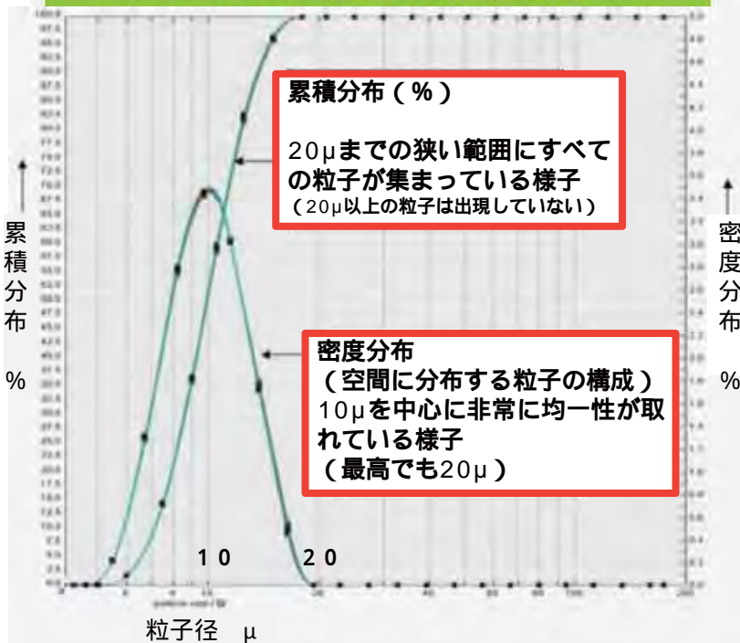
ノズル120mm前方の精度分布図
